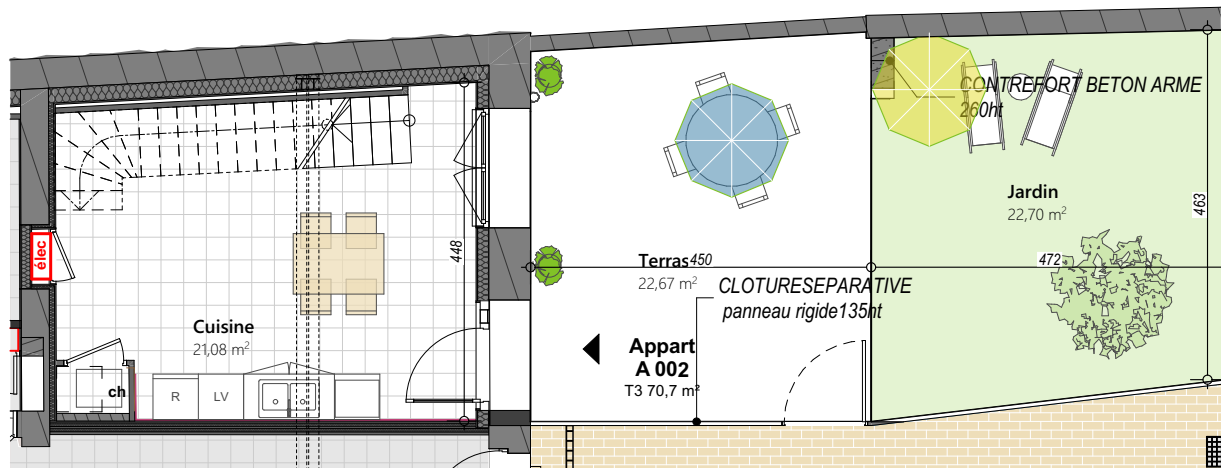
Plan du RDC
