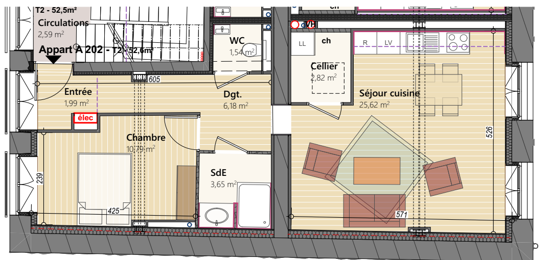
Plan du R+2
