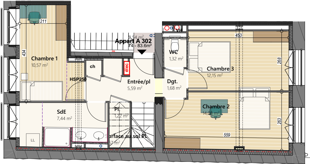
Plan du R+3
