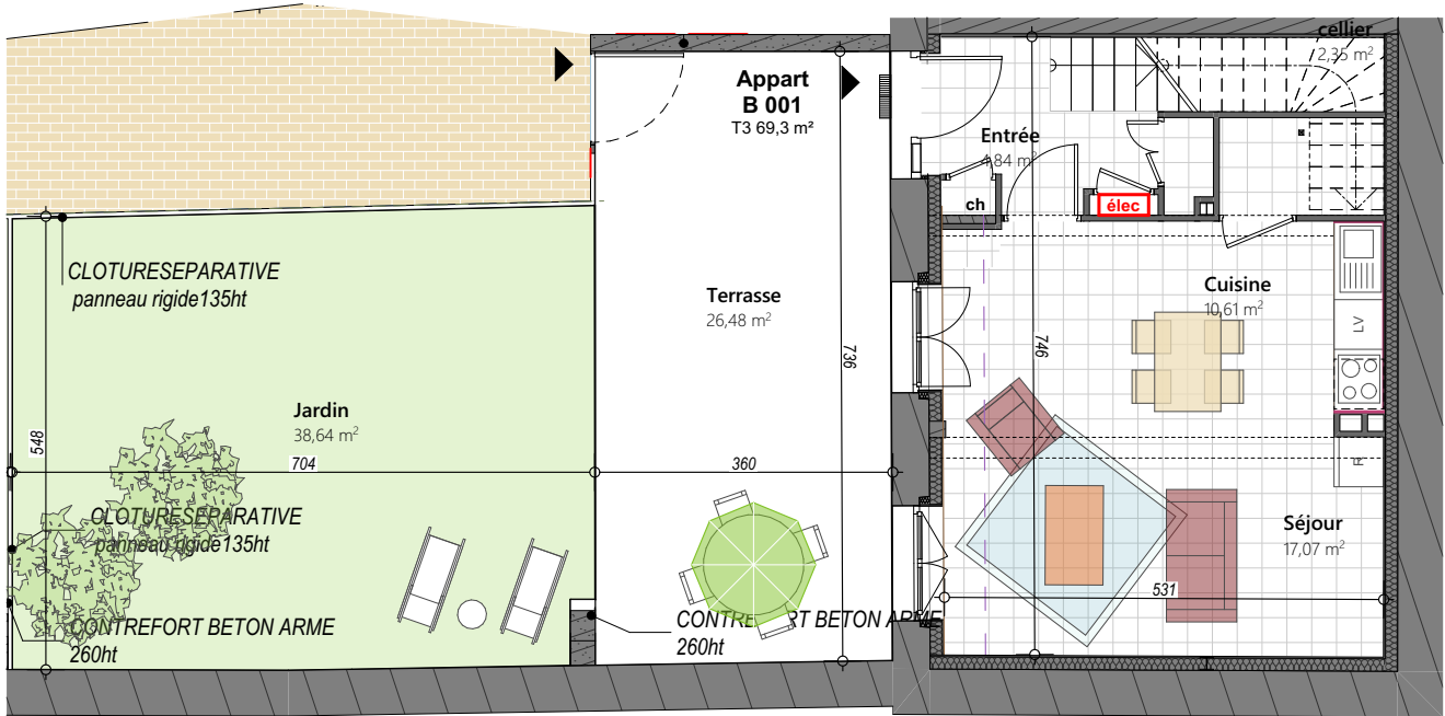
Plan du RDC
