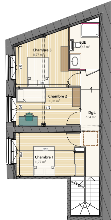
Plan du R+1
